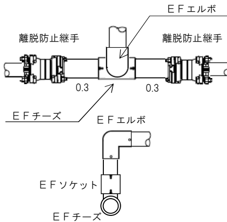
図ー4.6(e) 取付工 (30～40×50) 標準図
