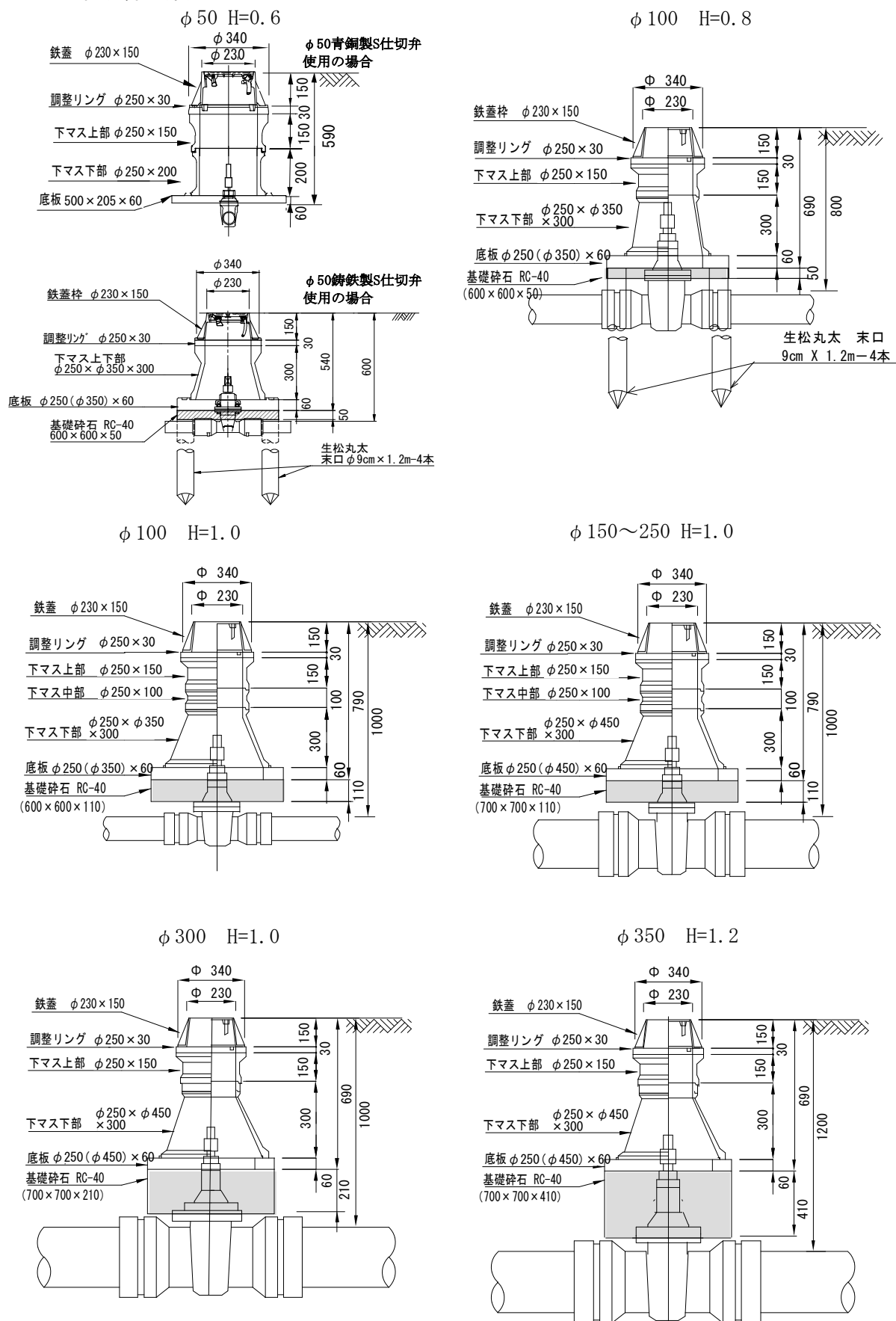
図-4.20 仕切弁室築造工標準図
