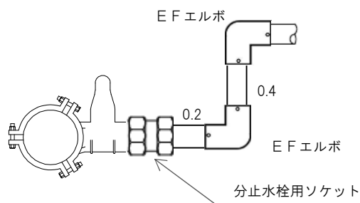
図-4.6(b) 取付工（75×50）標準図
