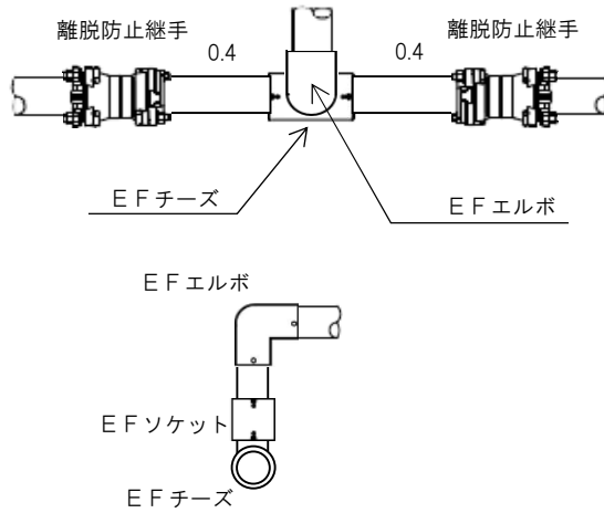
図ー4.6(d) 取付工 (50×50) 標準図
