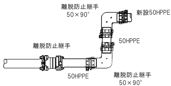
図ー4.7(a) 末端取付工 (50×50) 標準図
