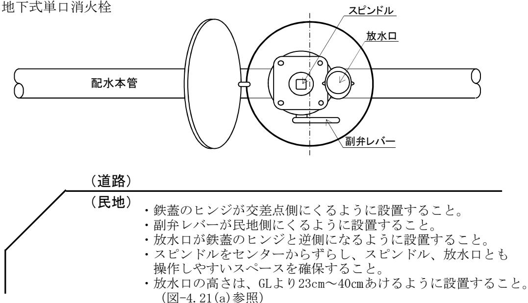
図-4.23 地下式単口消火栓設置標準図
