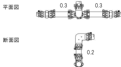
図-4.14 取付工 (30～40×50) 標準図
