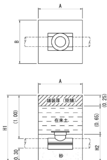
図-4.2(a) 不断水バルブ箇所 標準土工工事図
