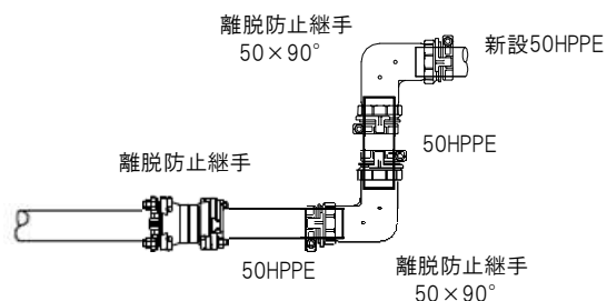
図-4.7(b) 末端取付工 (30～40×50) 標準図
