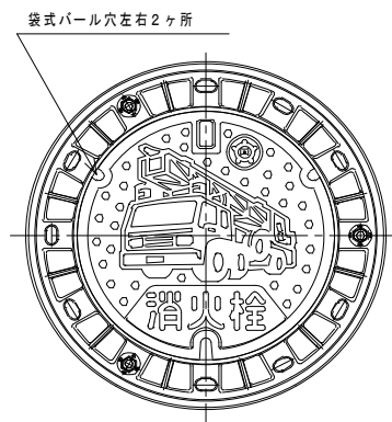
図-4. 21 (b) 消火栓鉄蓋標準図
