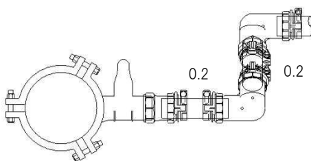
図-4.11 取付工(75×50)標準図
