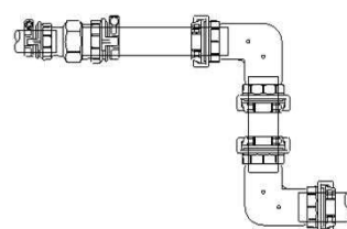
図-4.16 末端取付工 (30～40×50) 標準図
