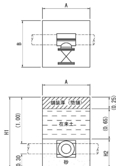
図-4.2(b) 不断水割T箇所 標準土工工事図
