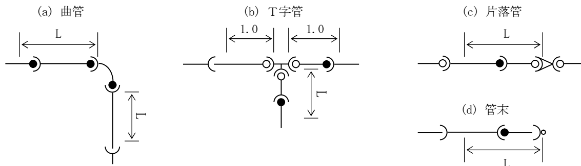
図-4.26 離脱防止金具取付け箇所
