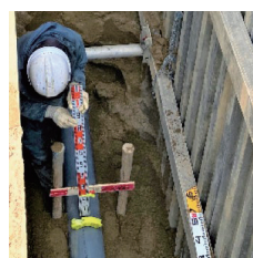
下水道管布設
