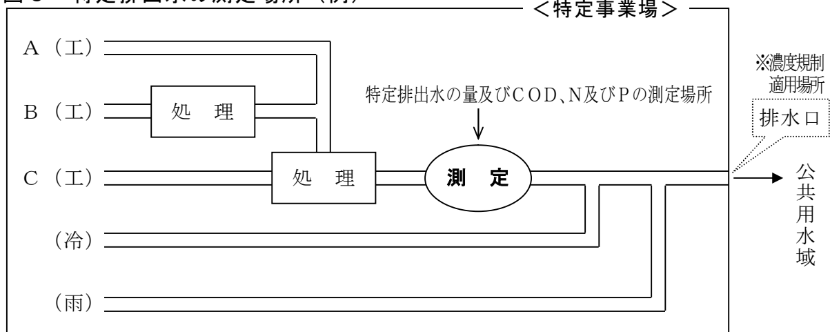
図 6 特定排出水の測定場所（例）
