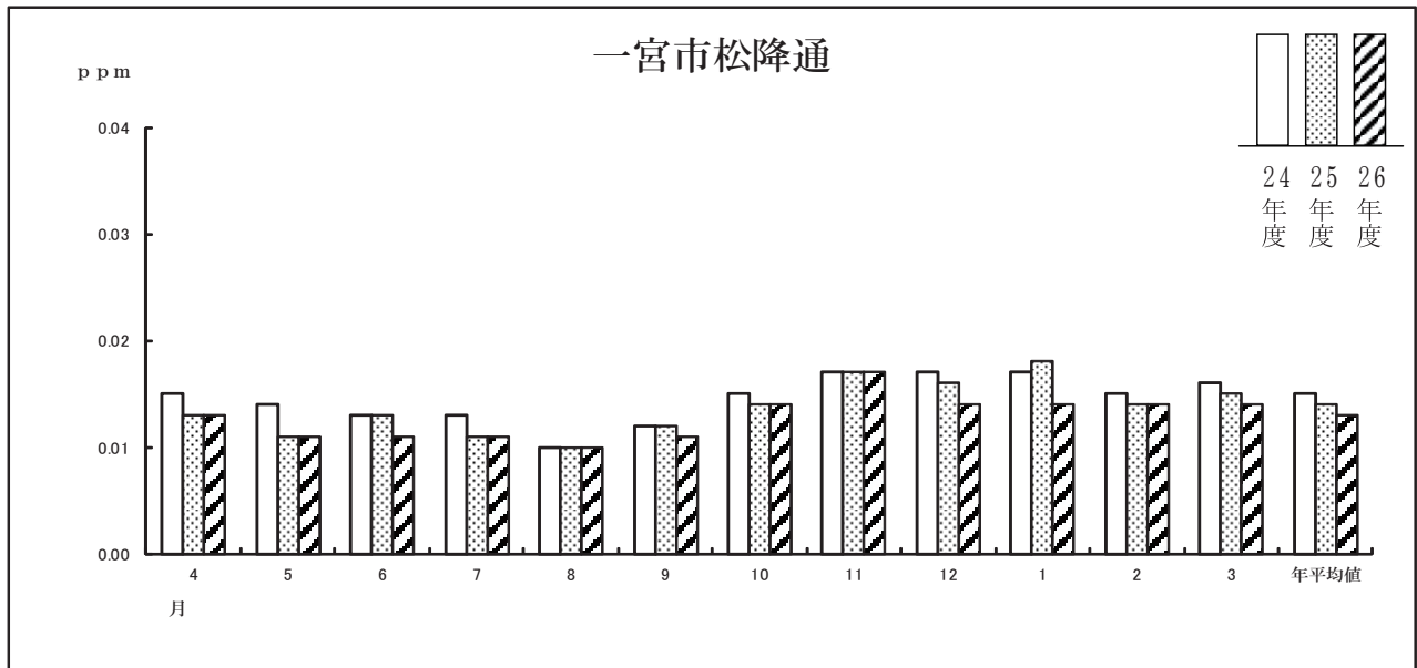
図6-3 NO 2 の推移
