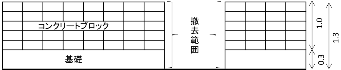
立面図
