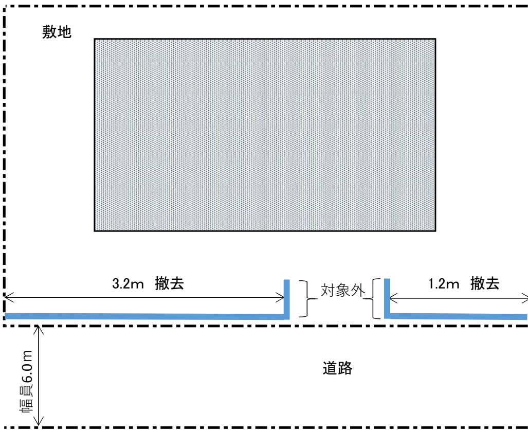
配置図
