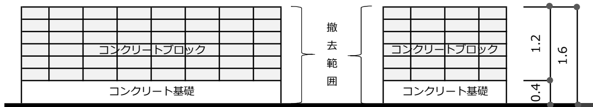
立面図
