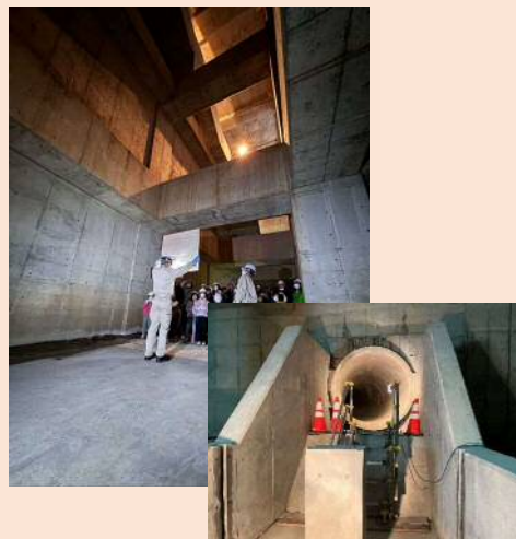
雨水管布設工事現場（管内部）
