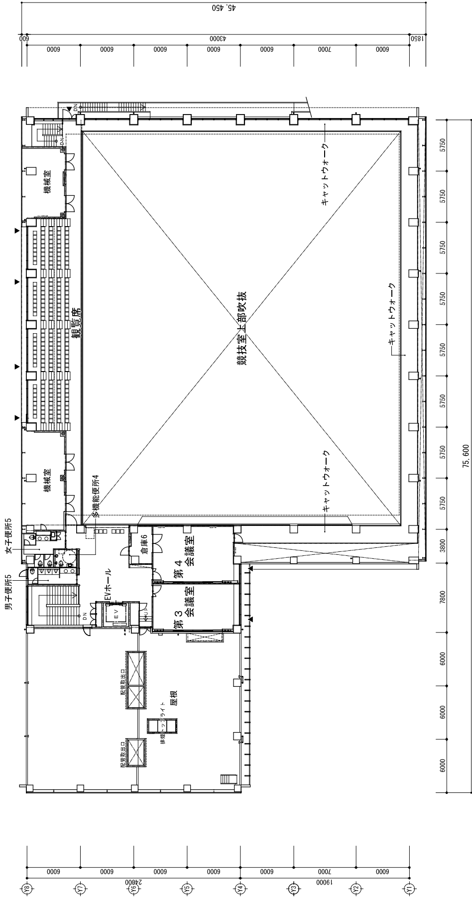
3階平面図
