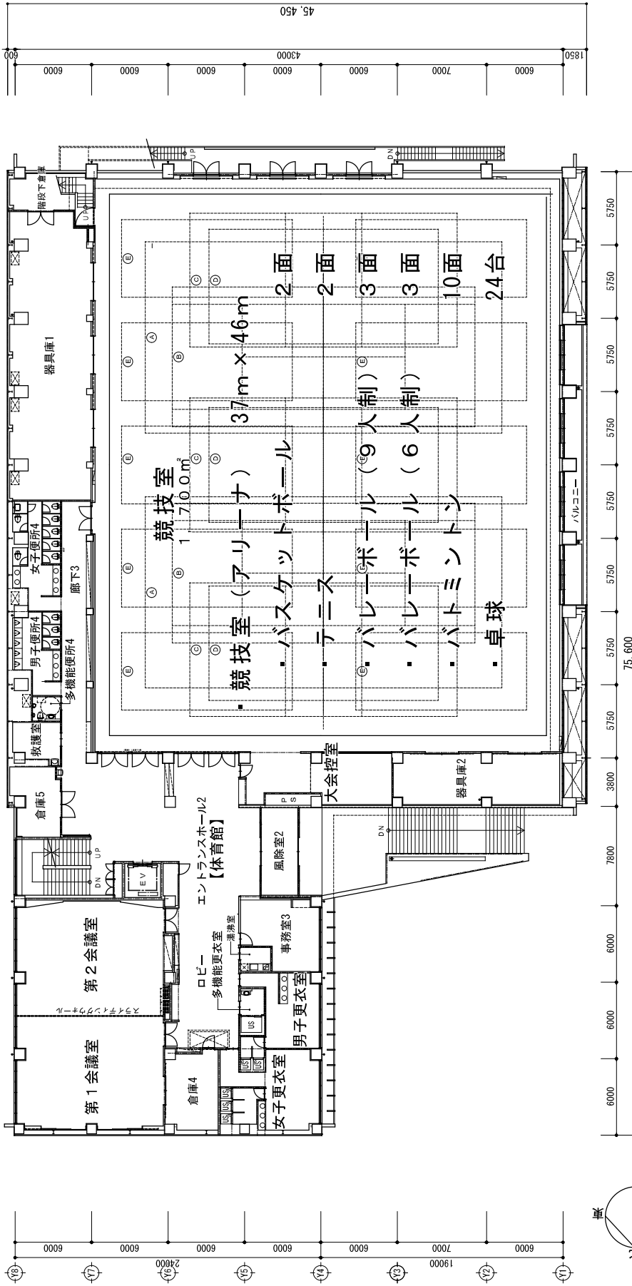
2階平面図
