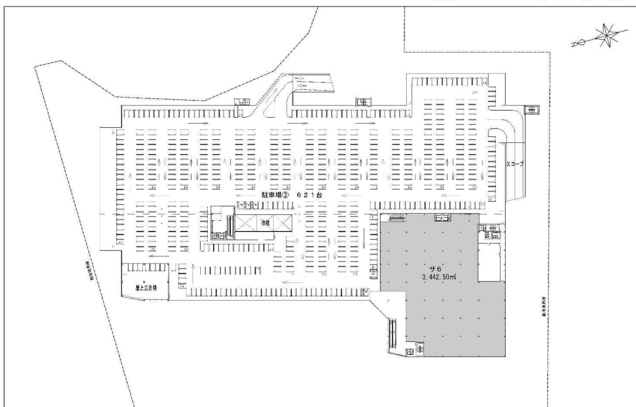
(仮称) ビバモール宮 3階平面図
