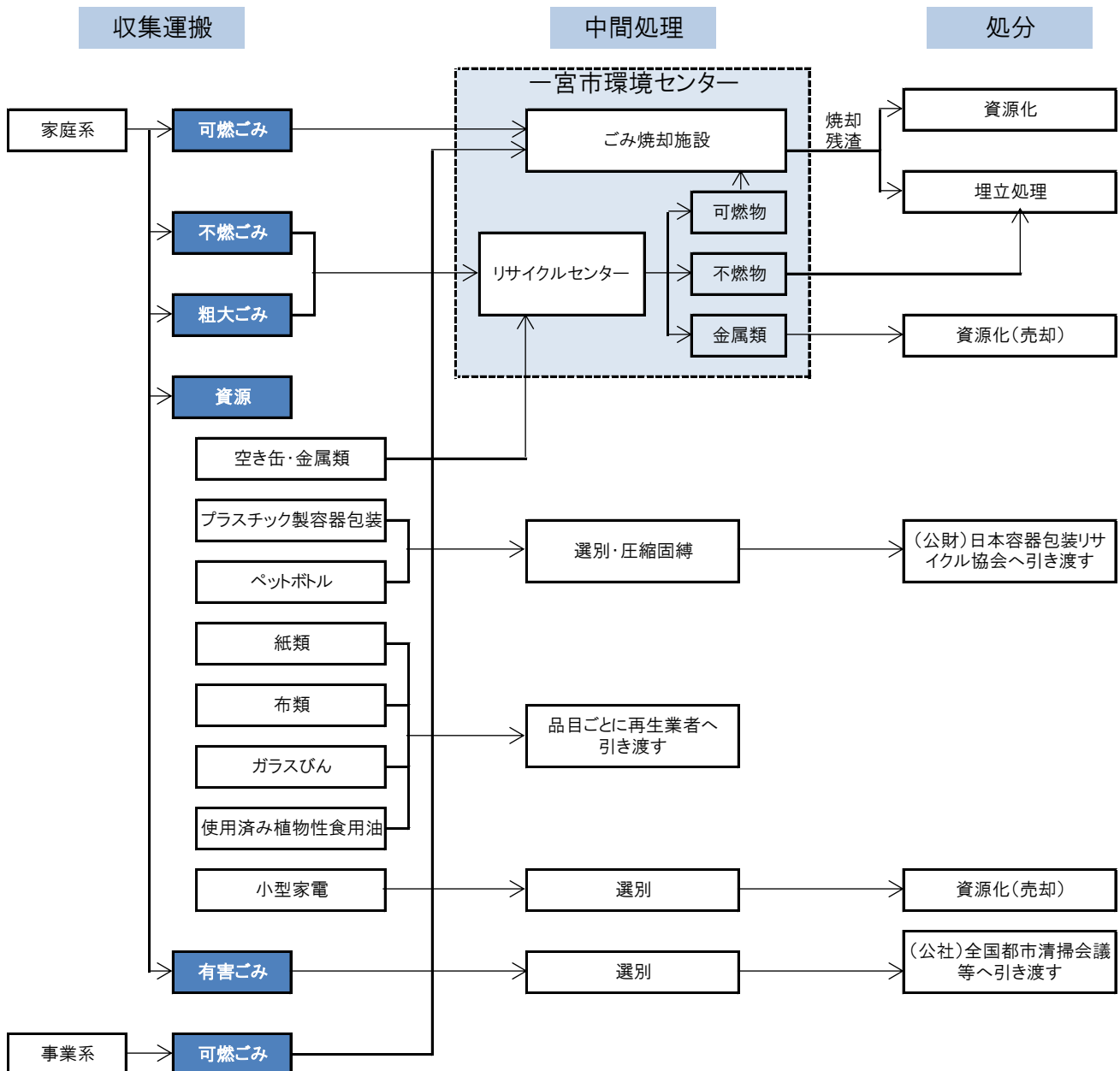
図 3-1 ごみ処理フロー
