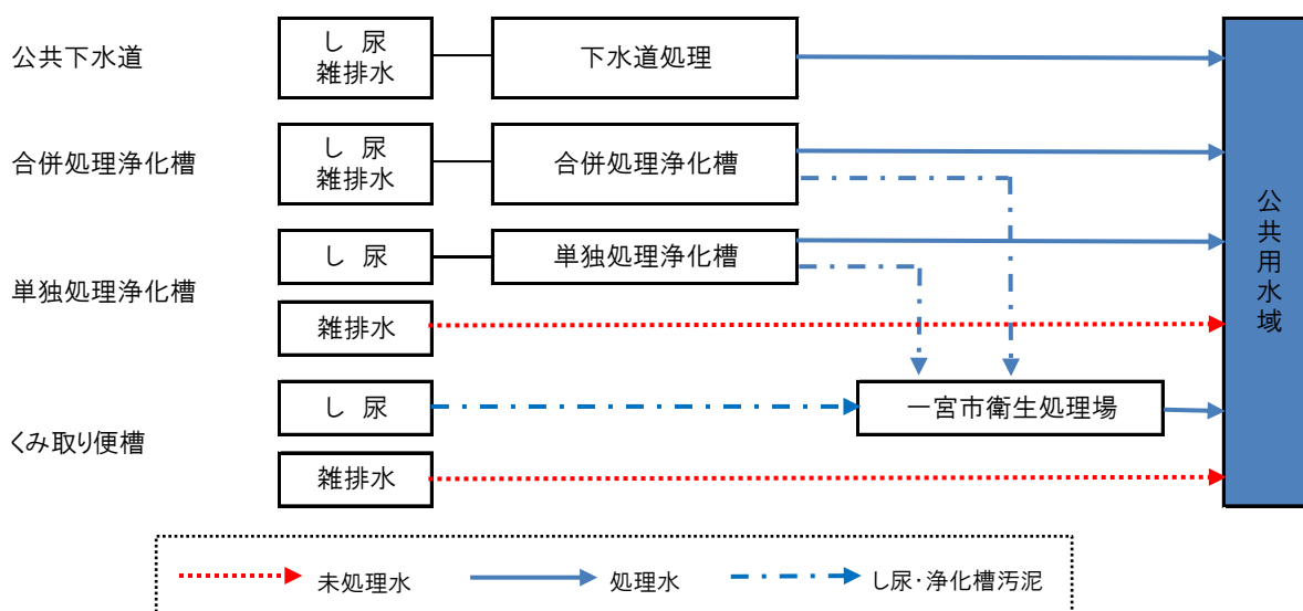
図 6-1 生活排水処理の概要
