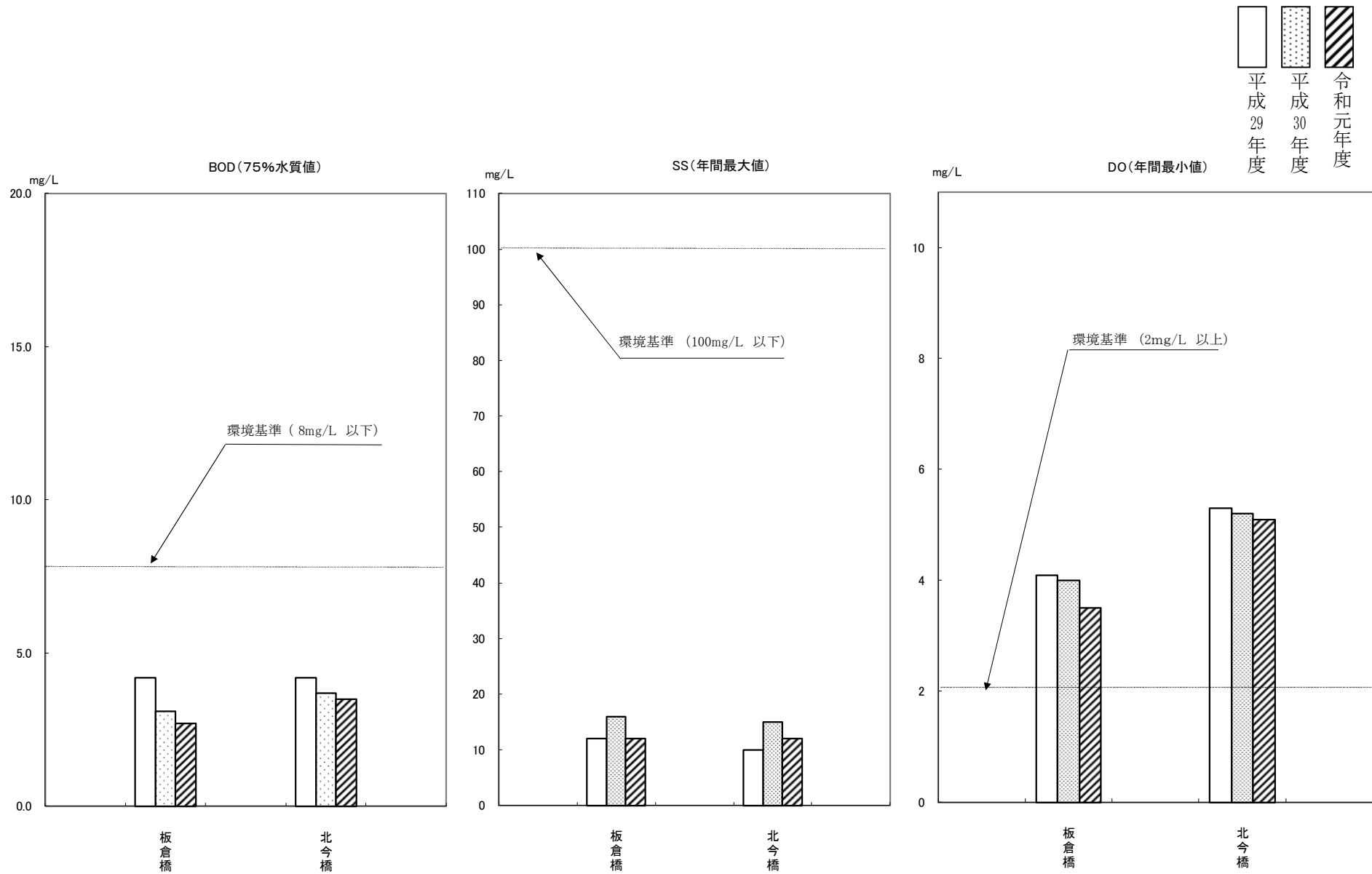
図7-1 日光川(環境基準点及び補助点)における水質経年変化
