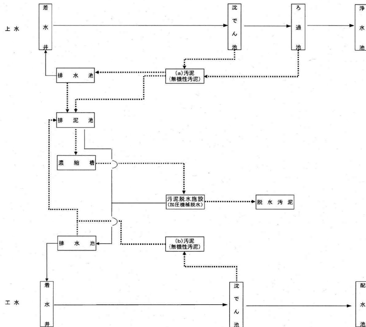
図4 排水処理フローシート
