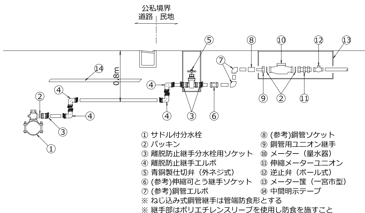
図 3-3 φ30mm～φ50mm 分水栓取出し標準図
