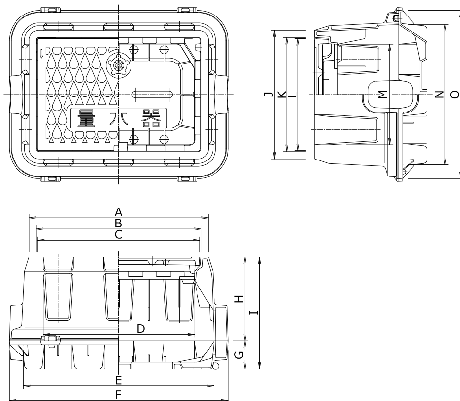
図 3-10 樹脂製メーター筐（φ13mm～φ40mm 用）
