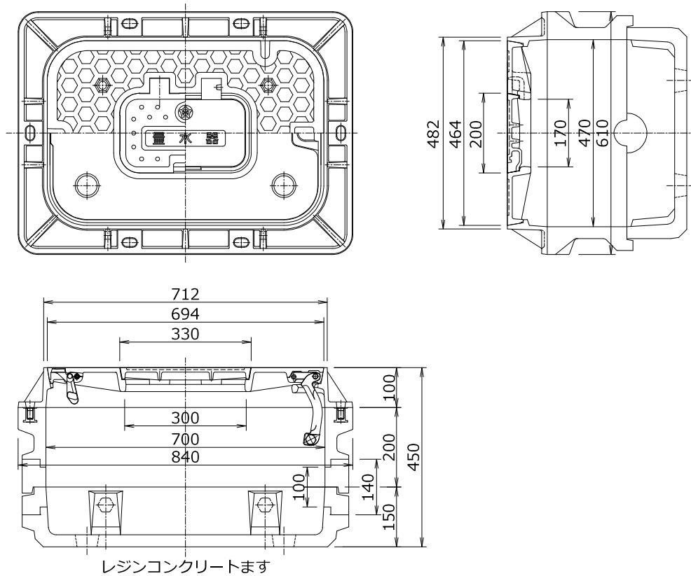
図 3-12 鋳鉄製メーター筐 (φ30mm・φ40mm 用)
