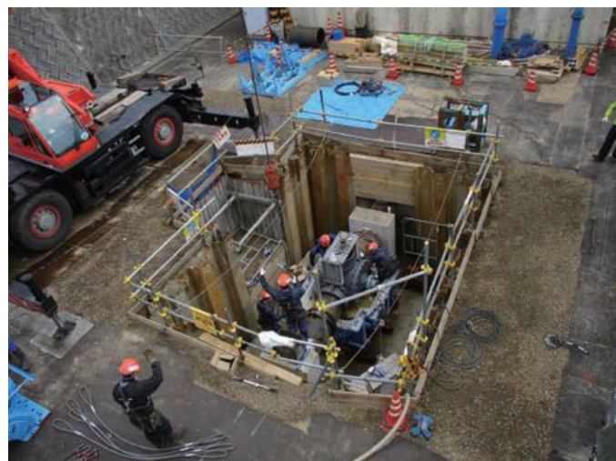
浄水場内の配水管布設
