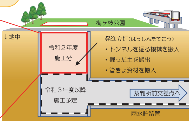
大和幹線雨水管布設工事の進捗イメージ
