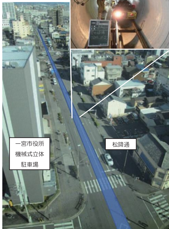
完成した本町幹線雨水管の位置及びイメージ
