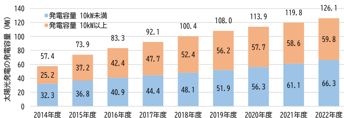
■FIT 認定太陽光発電の導入実績の推移
