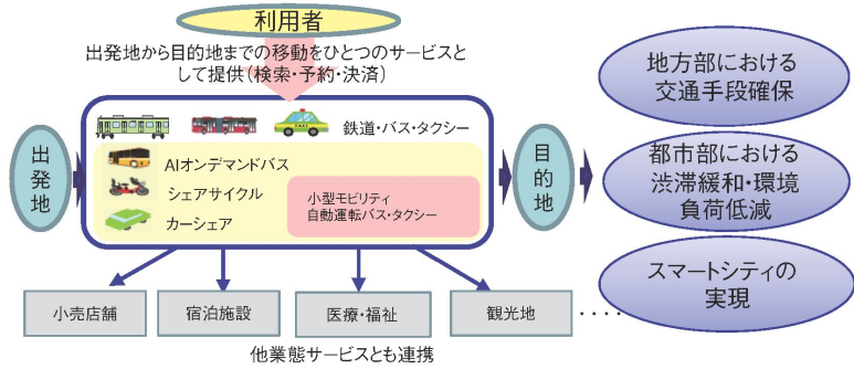
図 1.34 MaaS の概要
