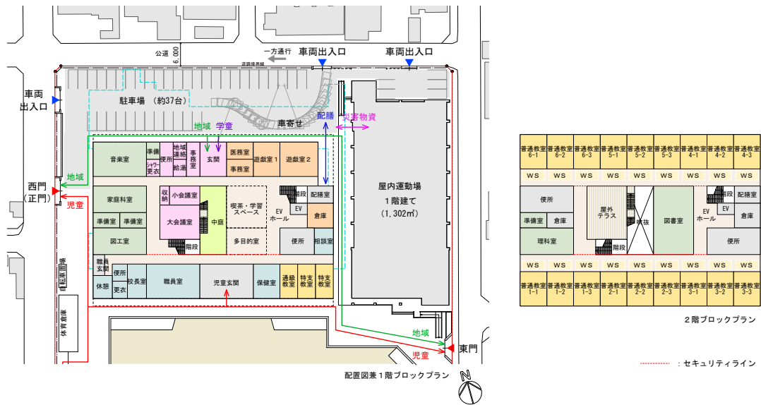
ブロックプランの検討（2階建て）
