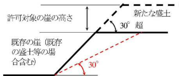
図1-3 崖の高さ（盛土）
