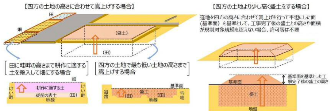
図 1-8 窪地における盛土規制要件の事例 イメージ図
