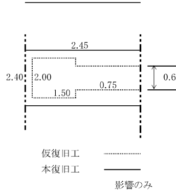
舗装展開図
