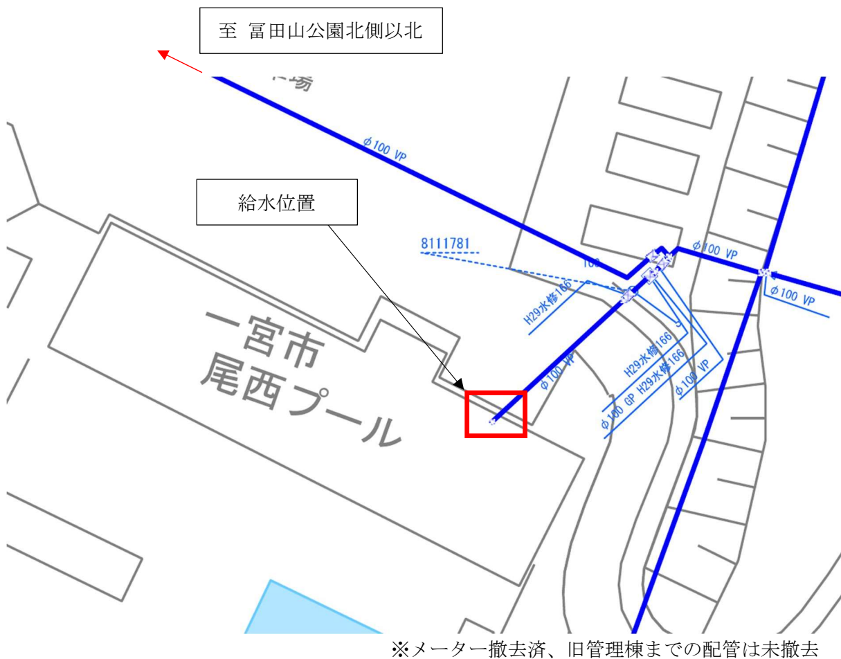
図4 給水位置図
