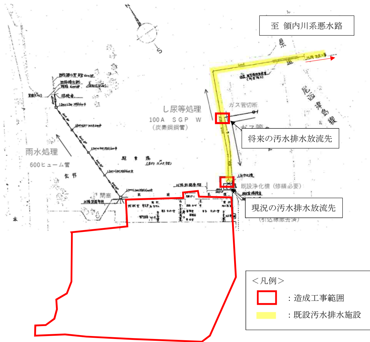
図5 雑排水処理水排水先位置図
