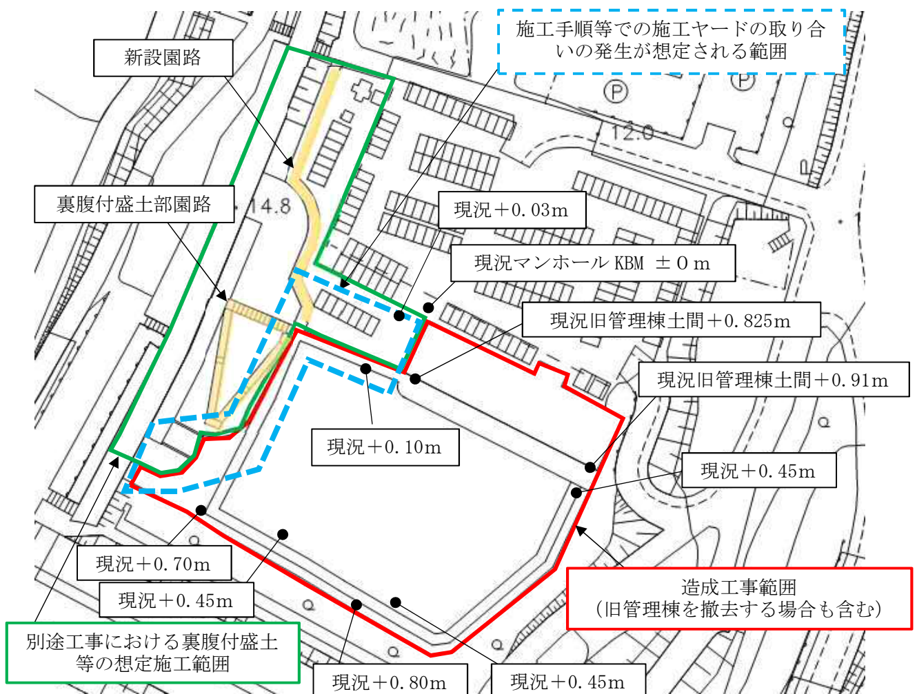
図1 施工ヤード関連位置図（イメージ図）
