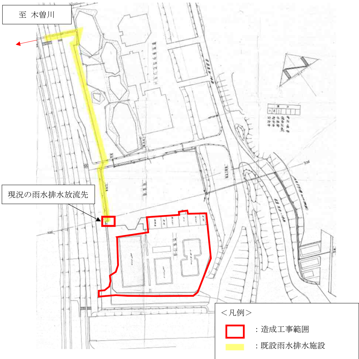
図3 既設の雨水排水施設
