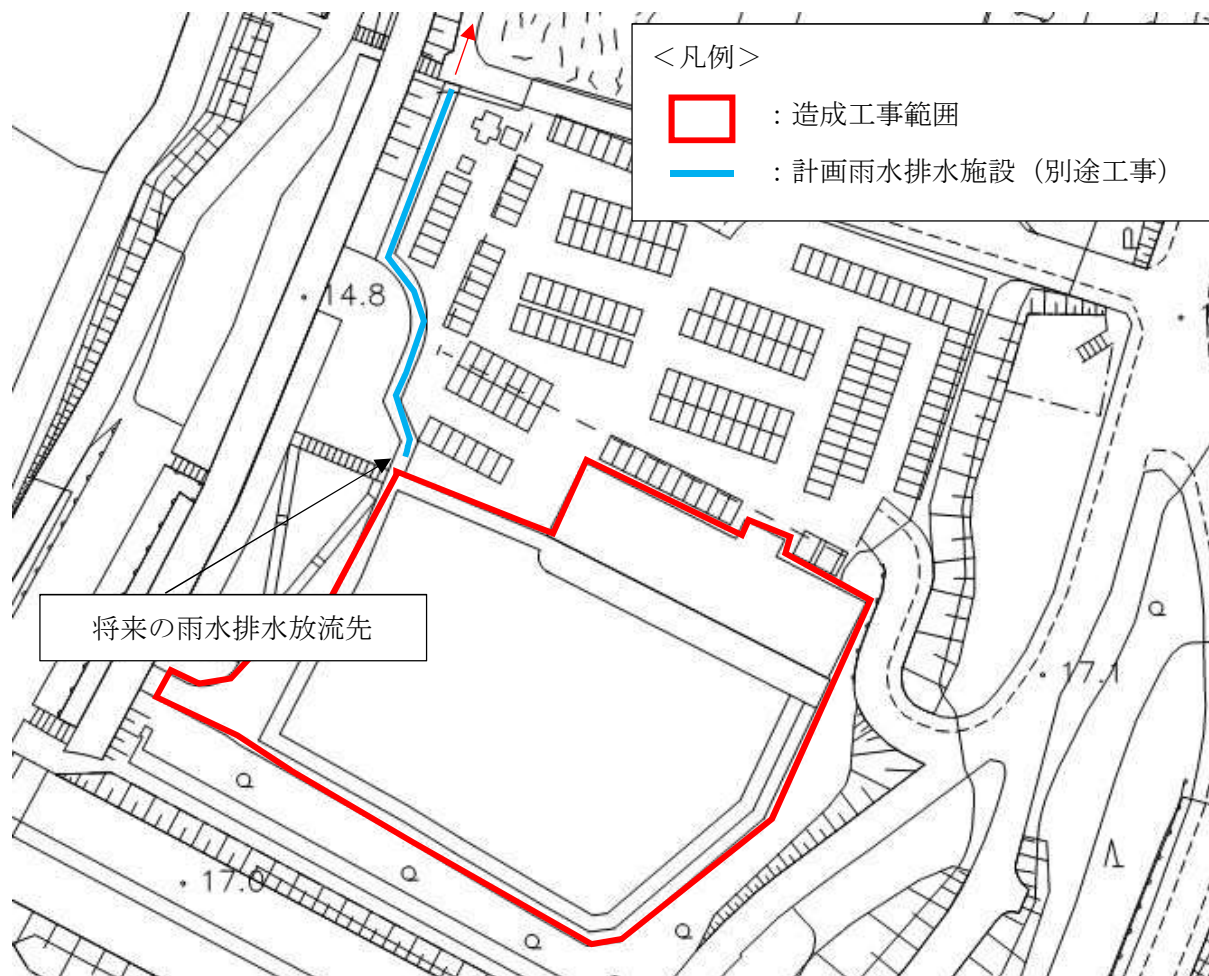
図2 放流先位置図
