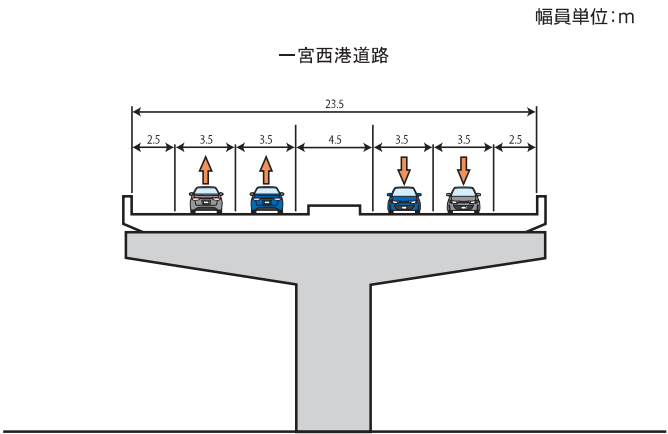
一宮西港道路の主な構造（標準的な横断面図）
