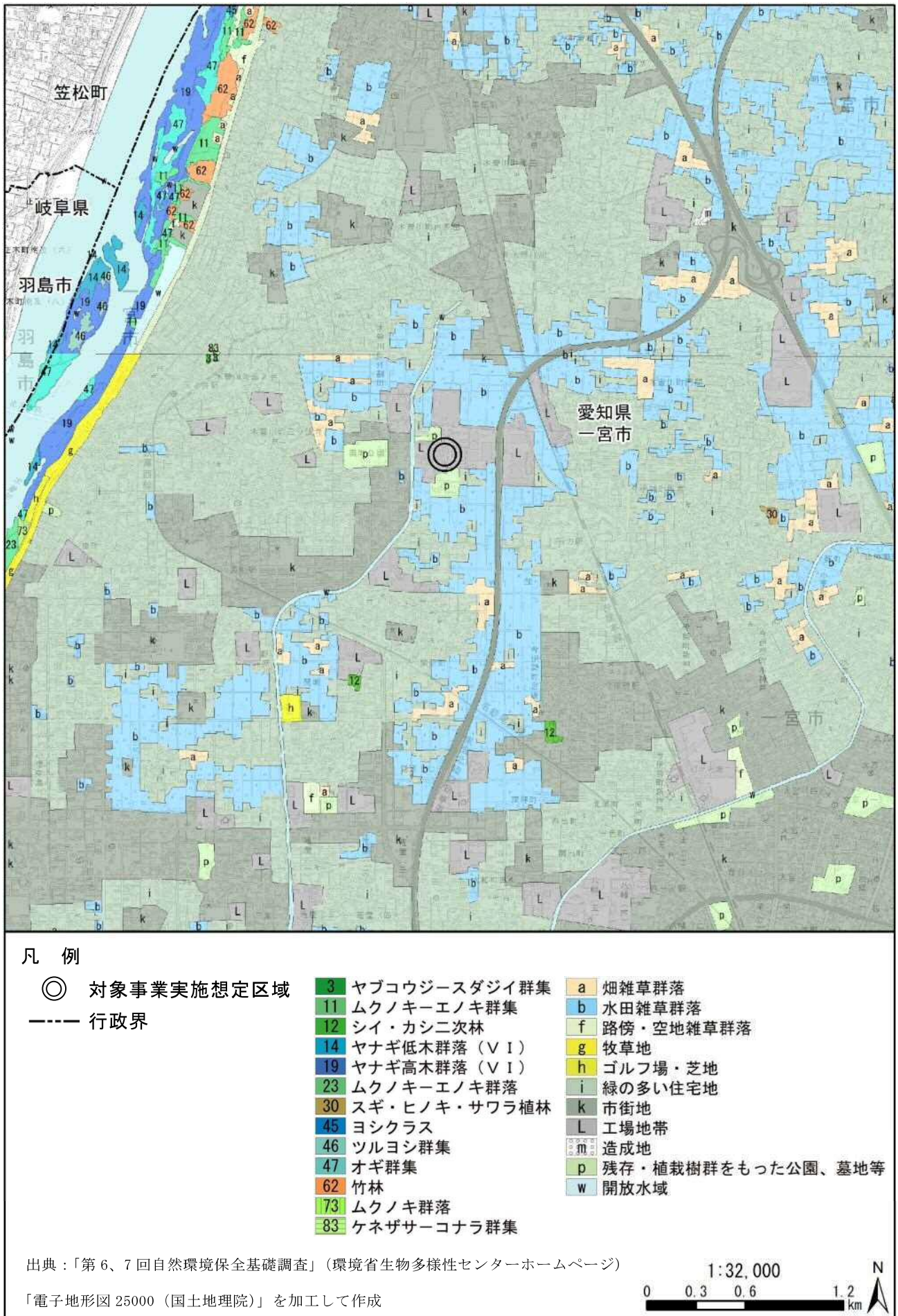
図 3.1.18 現存植生図
