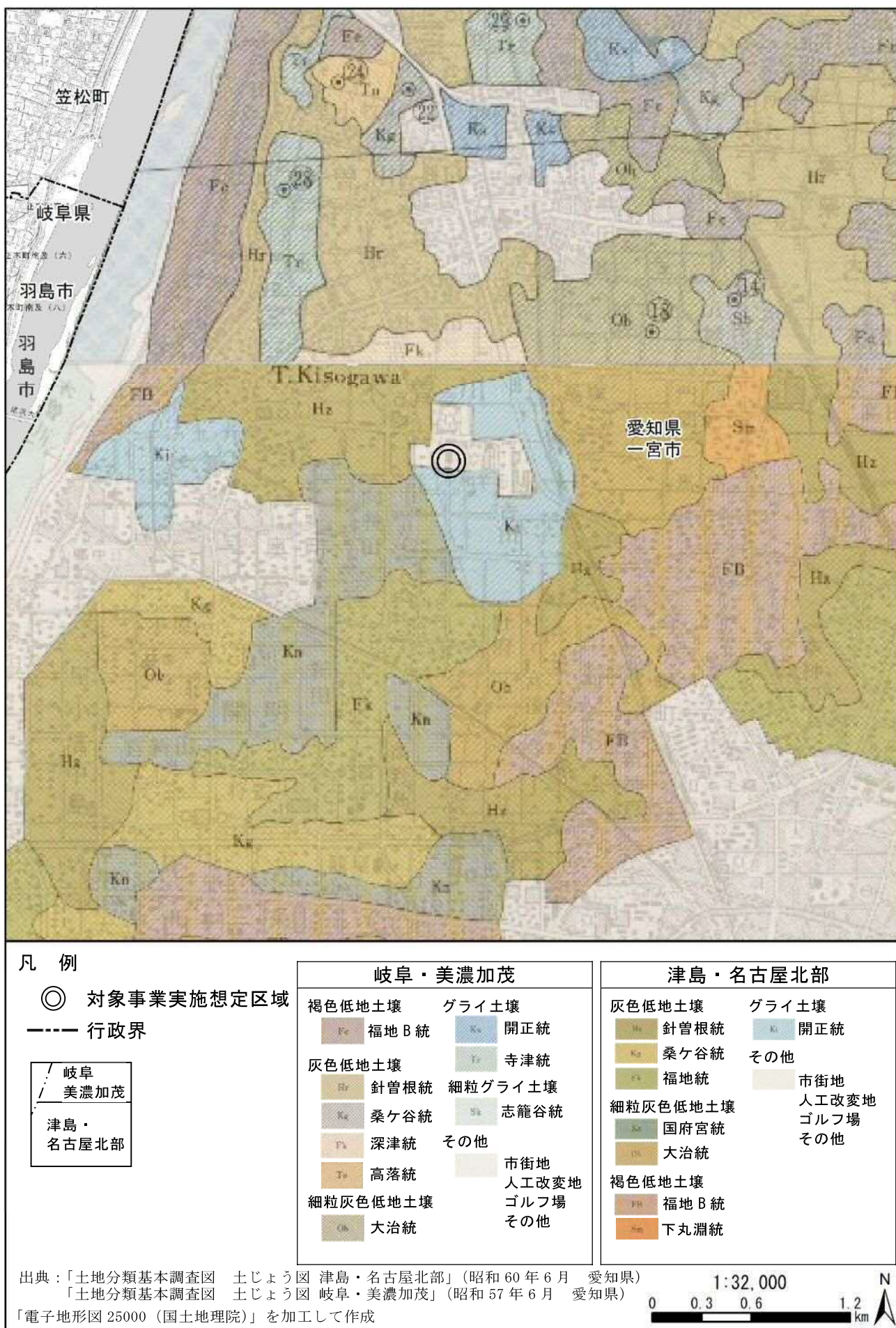
図 3.1.17 土壌図
