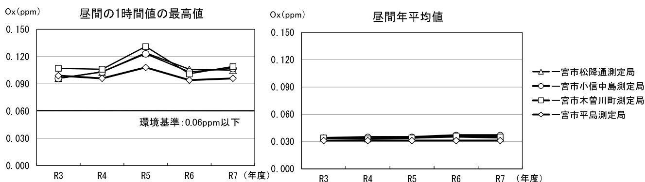
図 3.1.10 光化学オキシダントの経年変化
